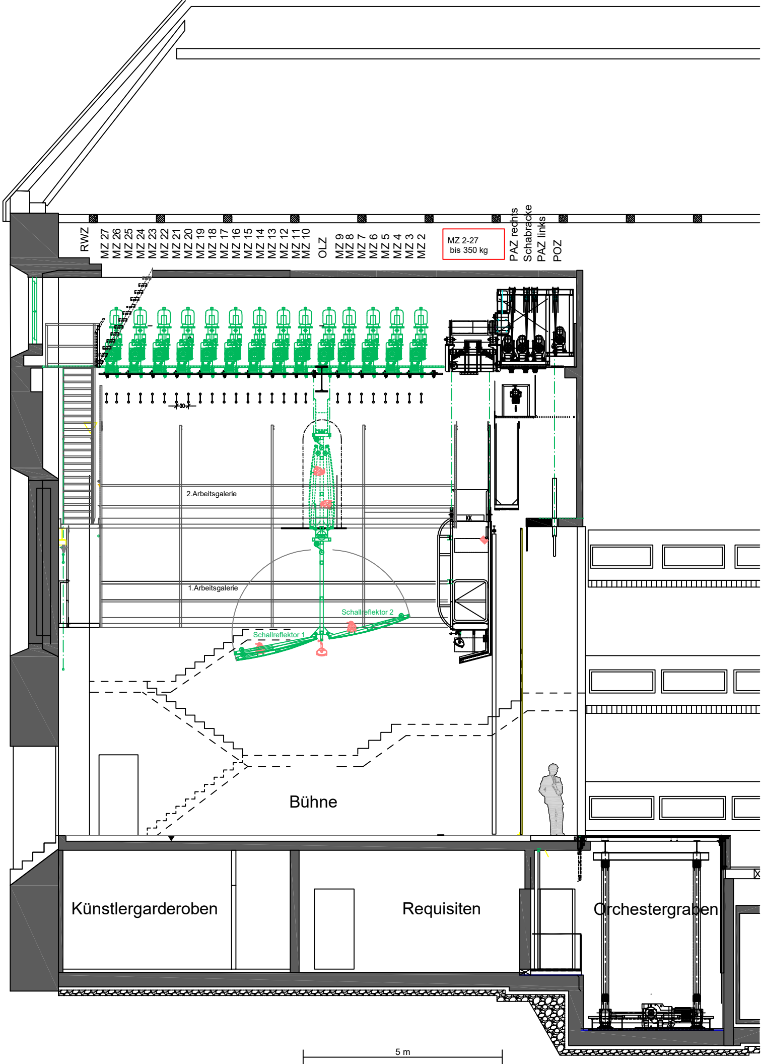
Schnitt Bühne
