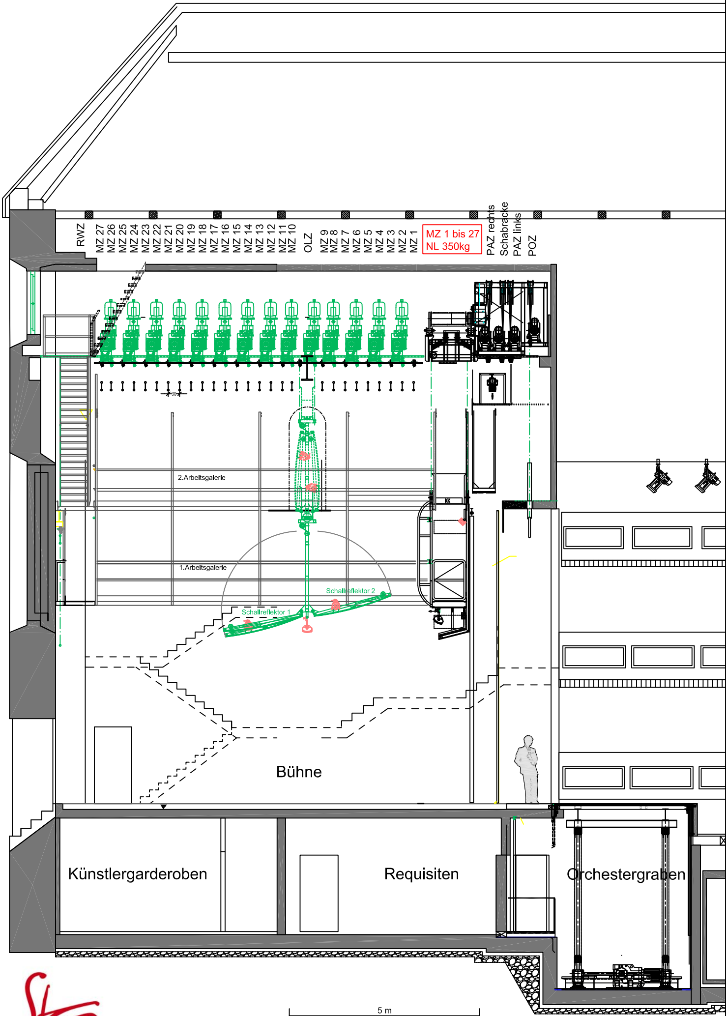
Schnitt Bühne
